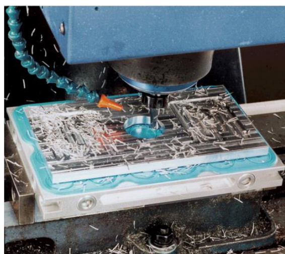
Fixação com placa de adaptação
